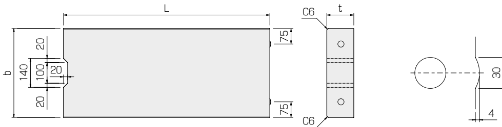
突起部詳細図
